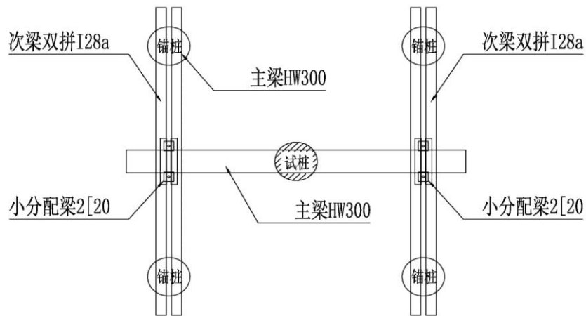
图 0-3 锚桩横梁反力装置示意图
