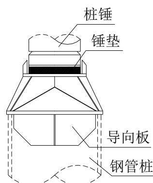
图 0-3 钢管桩锤击沉桩吊钟式替打示意图
