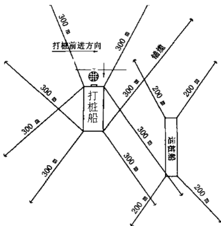
图 0-2 打桩船与驳船抛锚定位示意图
