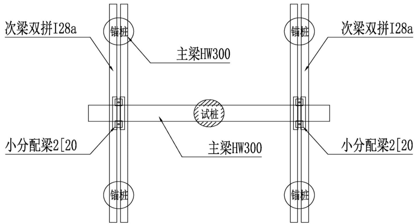
锚桩横梁反力装置示意图
