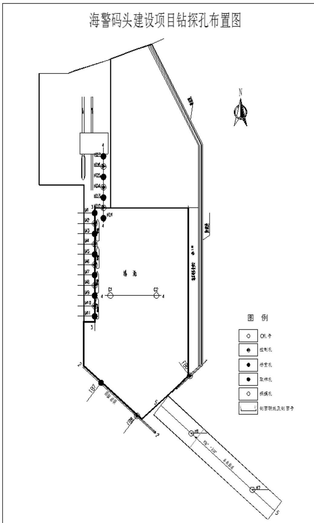
图 4.1-3 钻孔平面布置图
