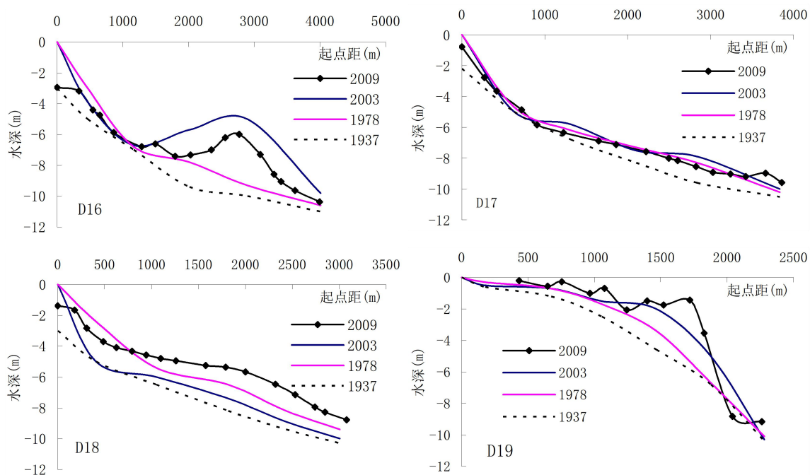
5.2-4 大范围海域断面水深对比
