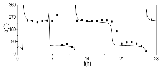
S6 测站实测与计算流向比较
