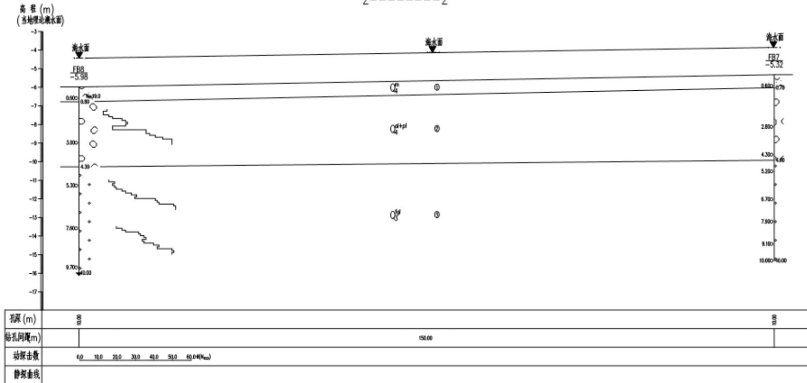
图 4.1-4 2-2' 工程地质剖面图
