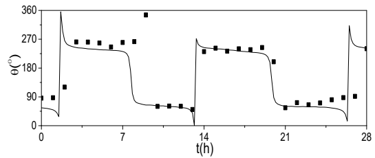
S5 测站实测与计算流向比较
