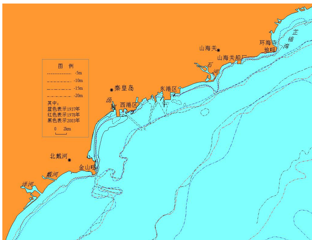
图 5.2-2 1937~2003年大范围海图等深线变化
